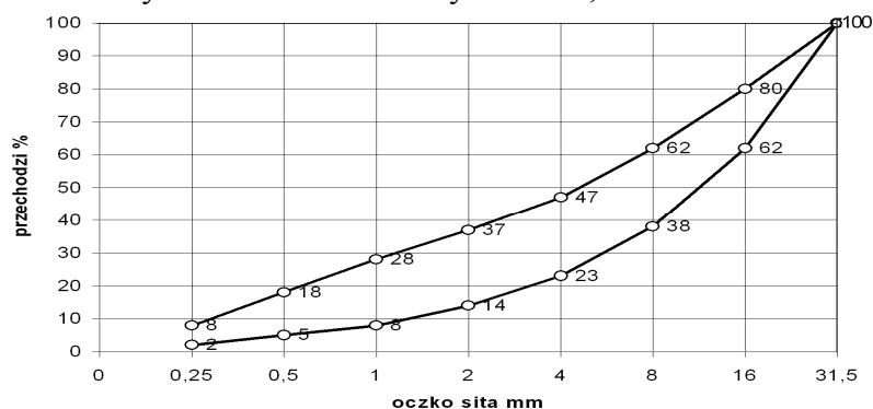
Rysunek 1. Graniczne krzywe uziarnienia kruszywa 0÷31,5 mm
