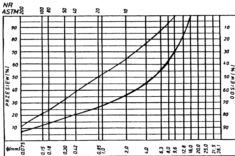
Tablica 4. Wymagania wobec mieszanek mineralno-asfaltowych oraz warstwy ścieralnej z betonu asfaltowego
