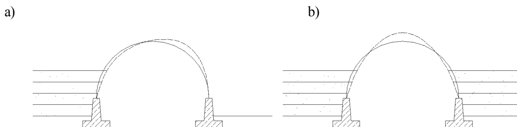
Rys. 4.4. Możliwe odkształcenia konstrukcji łukowej w przypadku: a) nieprawidłowego układania zasympki lub jej niesymetrycznego zagęszczania, b) braku kontroli odkształcenia przy symetrycznym układaniu zasympki, przy zbyt wysokim stopniu zagęszczenia.
