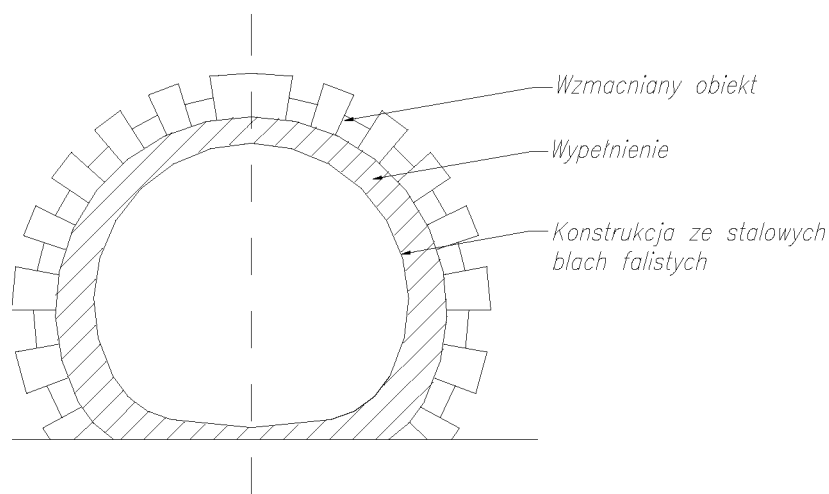
Rys. 5.1. Schemat obrazujący metodę reliningu.
