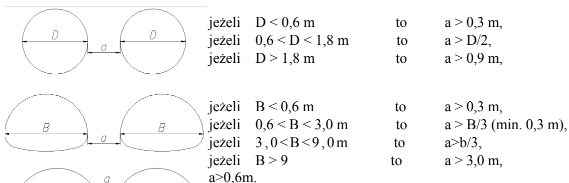
Rys. 3.1. Minimalne odległości pomiędzy konstrukcjami z blach
