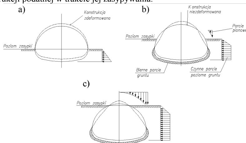
Rys. 4.5. Stan równowagi konstrukcji podatnej w czasie jej zasypywania: a) zasypka poniżej linii maksymalnej rozpiętości; b) zasypka powyżej linii maksymalnej rozpiętości; c) zasypka w pobliżu klucza konstrukcji.
