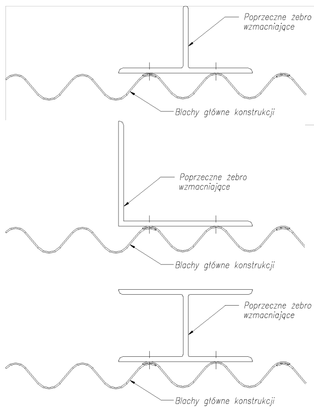
Rys. 3.14. Poprzączne żebra wzmacniające wykonane z kształtowników metalowych.
