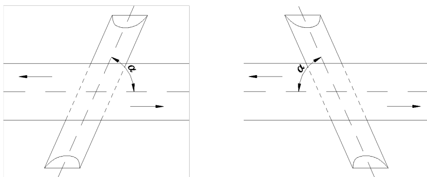
Rys. 3.16. Kąt skrzyżowania obiektu z osią drogi. Jest to zawsze kąt < 90^\circ niezależnie od kierunku kilometraża drogi.
