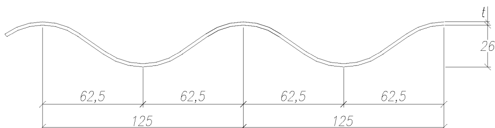
Rys. 2.5. Przykład profili fal o wymiarach: a) 68x13 mm; b) 100x20 mm; c) 125x26 mm.
