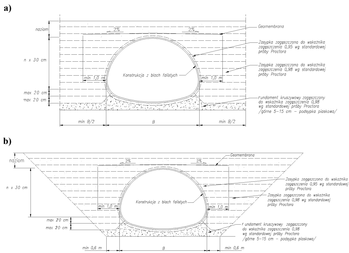
Rys. 4.3. Sposób układania zasypki wokół konstrukcji z blach falistych: a) nasyp b) wykop.
