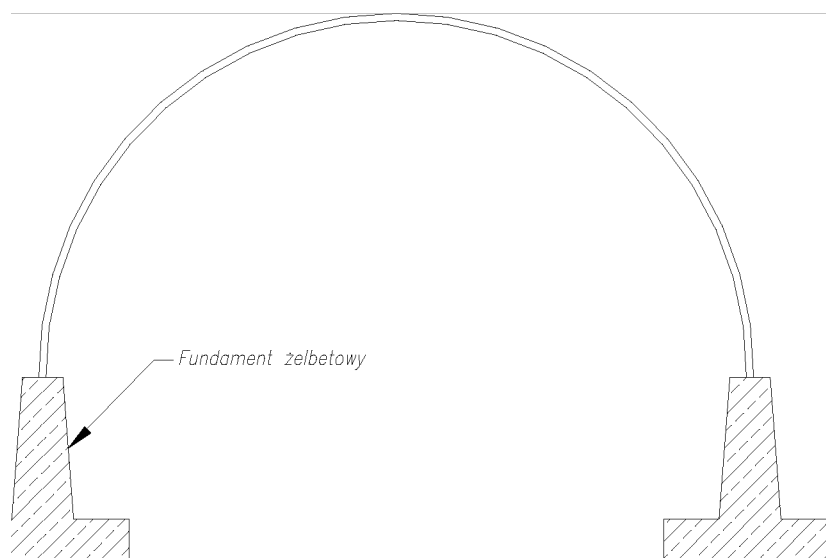
Rys. 3.2. Konstrukcja z blach falistych oparta na żelbetowym fundamencie.
