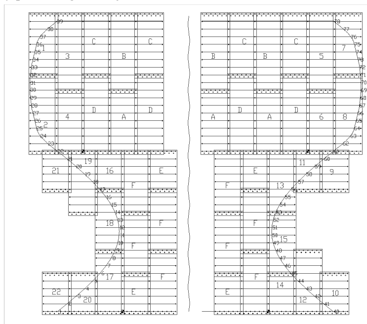
Rys. 4.2. Przykładowy rysunek montażowy.
