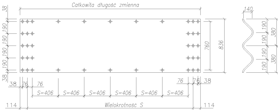
Rys. 2.4. Przykład arkusza blachy o profilu fali 380x140 mm.
