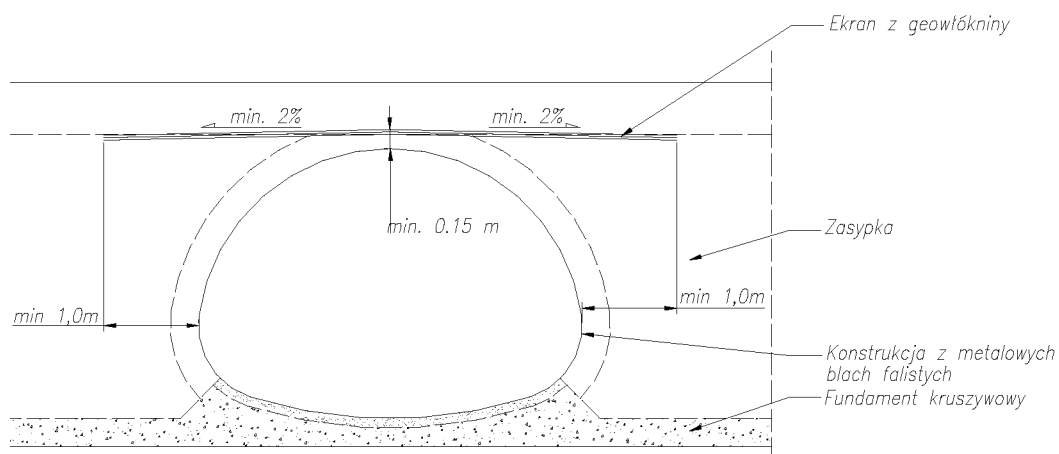
Rys. 4.7. Zabezpieczenie konstrukcji przed wodą opadową.
