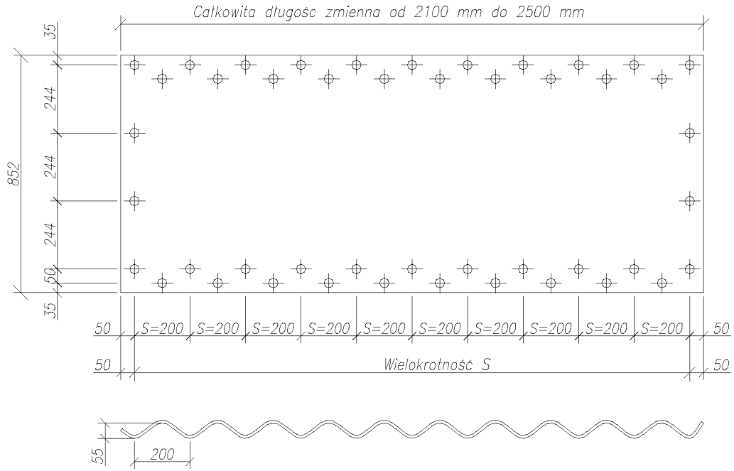
Rys. 2.3. Przykład arkusza blachy o profilu fali 200x55 mm.
