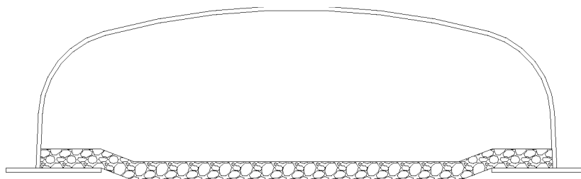
Rys. 3.5. Wzmocnienie dna ciekę geosyntetykami i z wypełnieniem materiałem skalnym.
