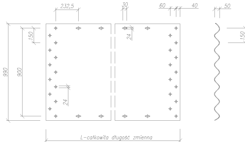
Rys. 2.2. Przykład arkusza blachy o profilu fali 150x50 mm.
