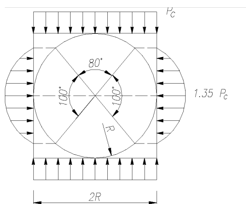
Rys. 3.8 a. Rozkład parcia gruntu na konstrukcję podatną wg Marstona-Spanglera.
