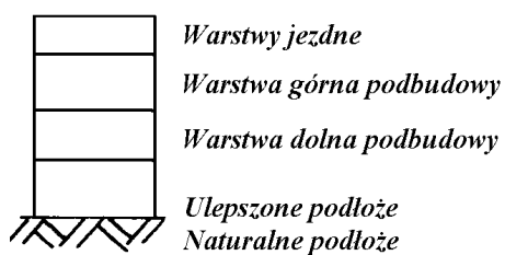
Rys. 4. Przykładowe wybrane konstrukcje nawierzchni utwardzonego pobocza z kruszywą łamaną niezwiązaną
