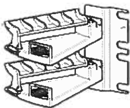
Rys 4. Organizator pionowy z kontrolą zgięcia, Hi-D
