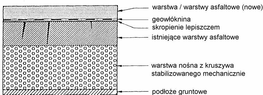
Rys. 2. Wzmocnienie nawierzchni asfaltowej bez warstwy profilującej
